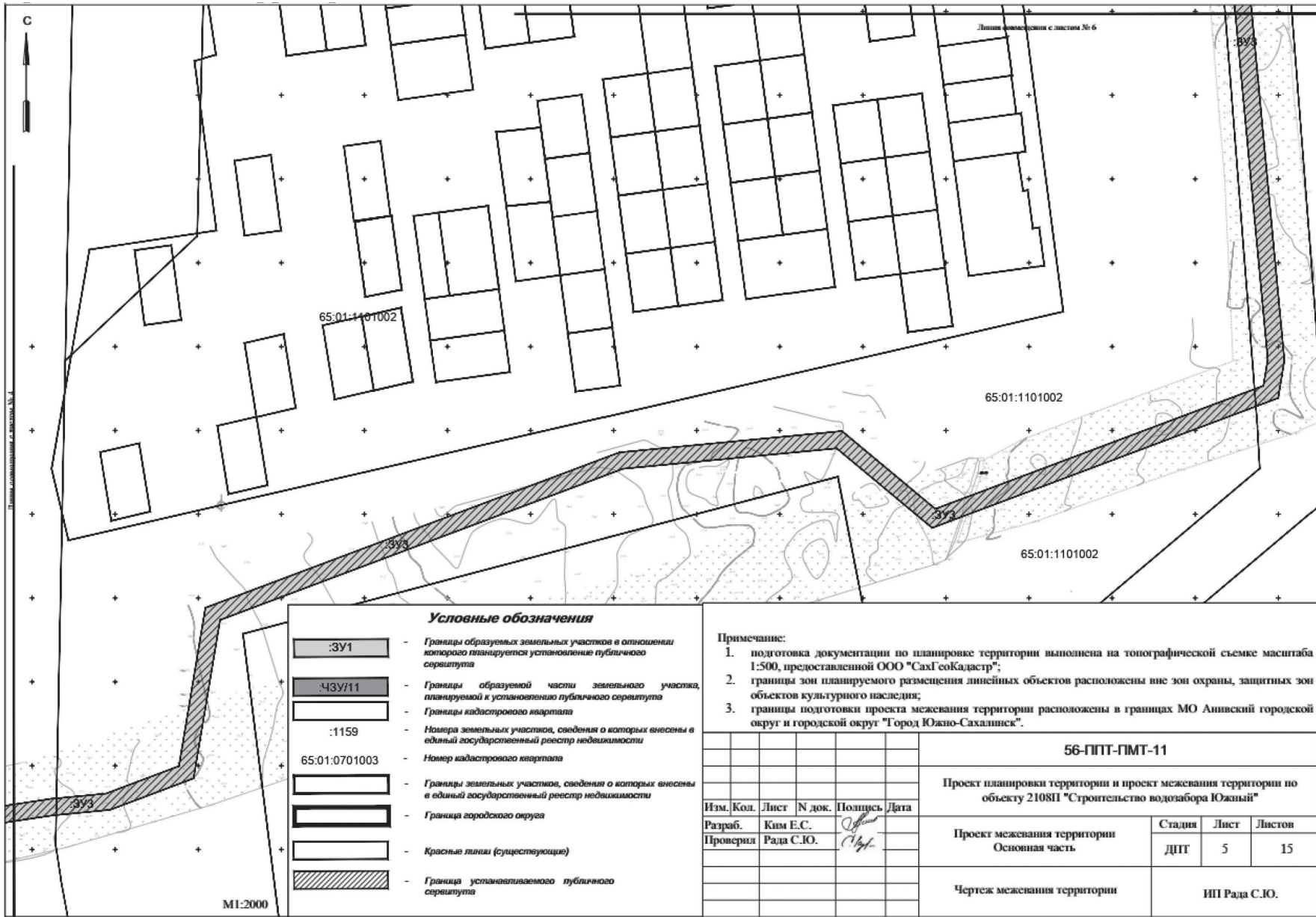
Чертеж межевания территории
