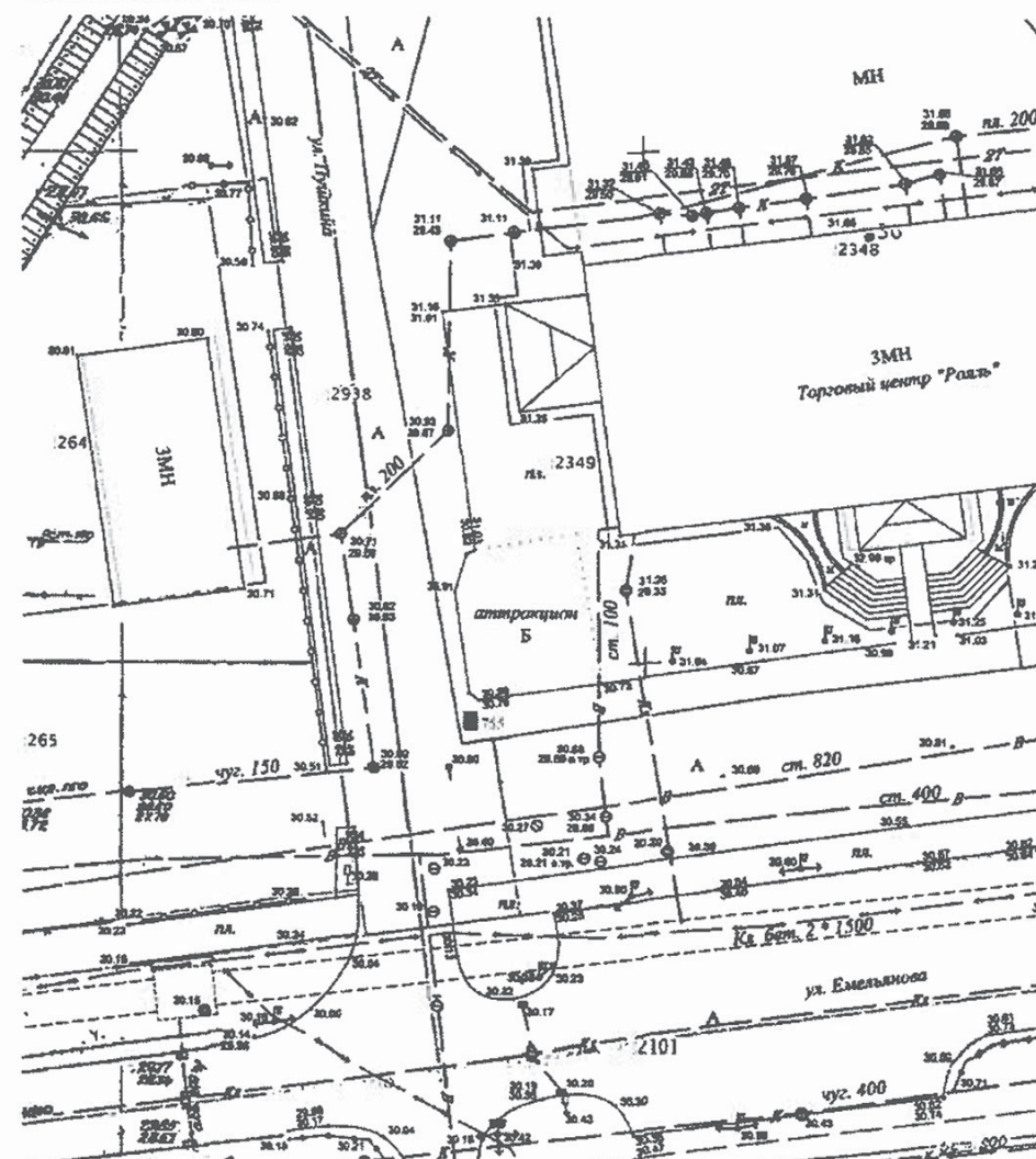
Топосъемка М 1:500
