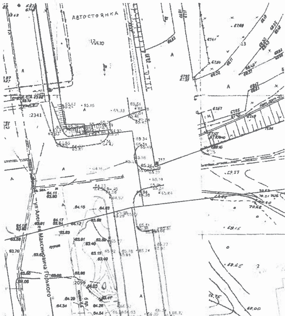
Топоусьмка М 1:500
