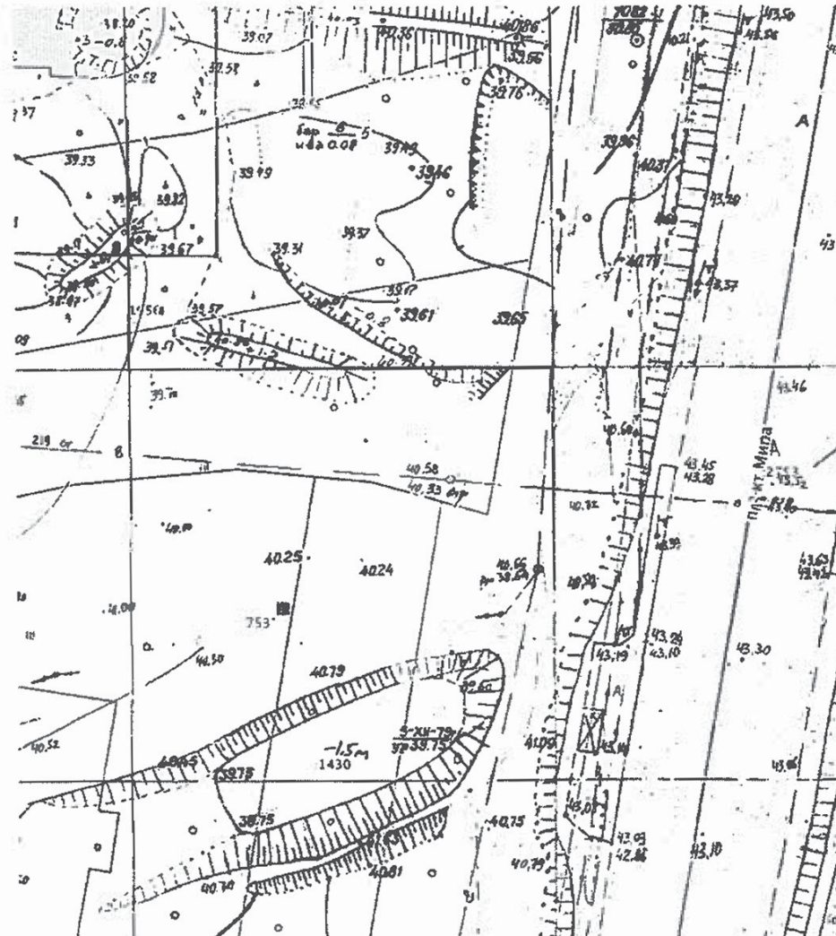
Топосъемка М 1:500
