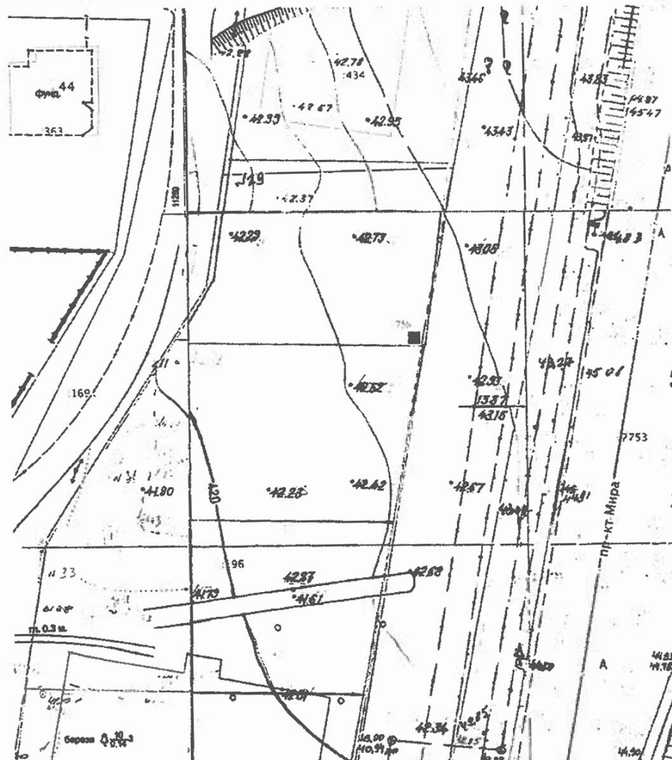
Топоусьмка М 1:500
