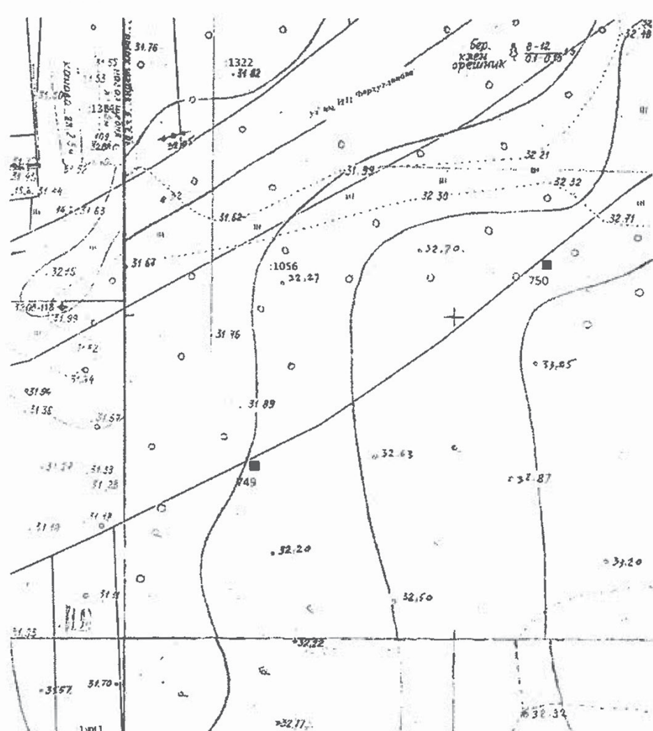
Топосъемка М 1:500
