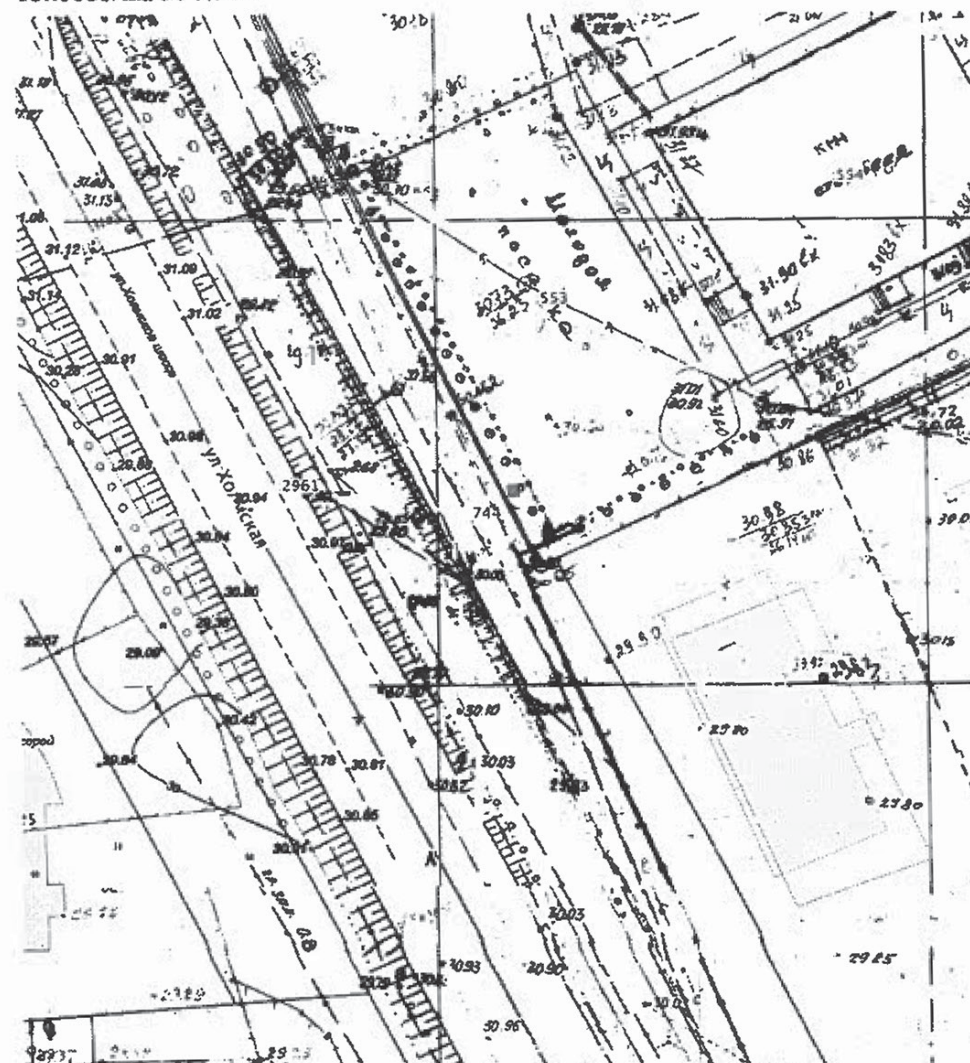
Топосъемка М 1:500
