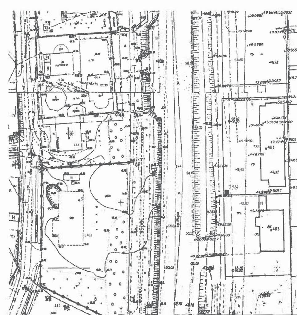
Топосъемка М 1:500
