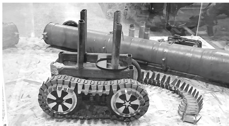
» Радиоуправляемое наземное устройство подрыва опорных пунктов противника, изготовленное нашими бойцами
