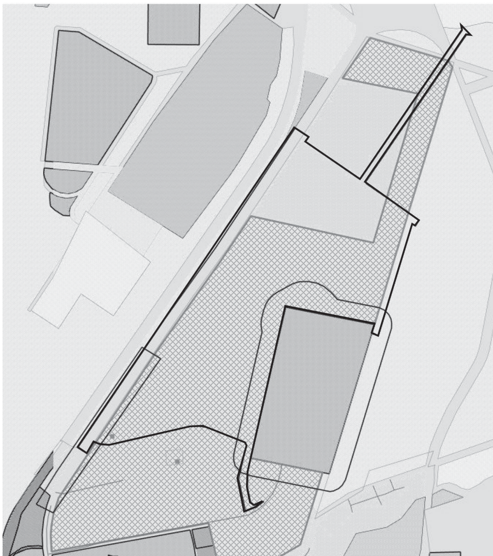
— границы проектирования
