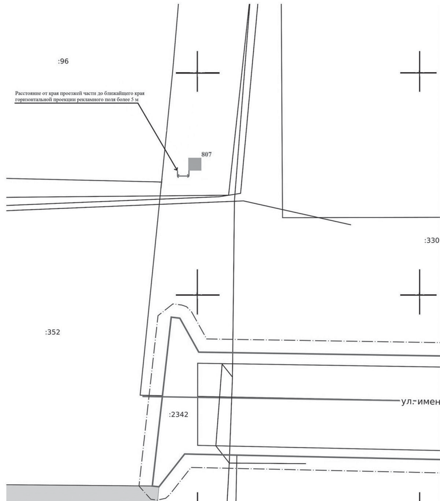
Топосъемка М 1:500
